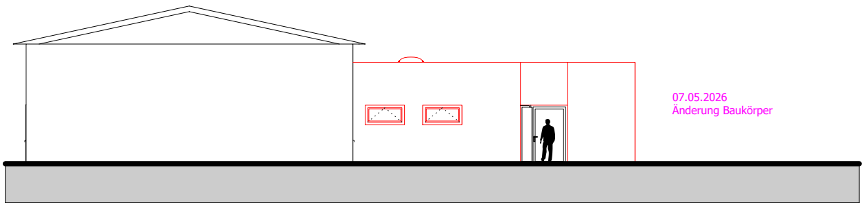
Ansicht West
